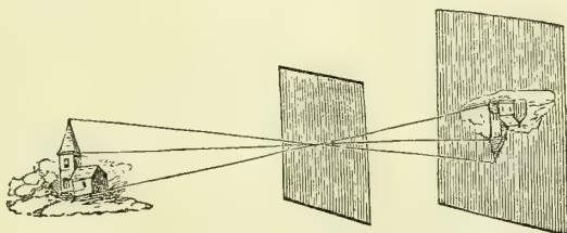
Camera Obscura.
